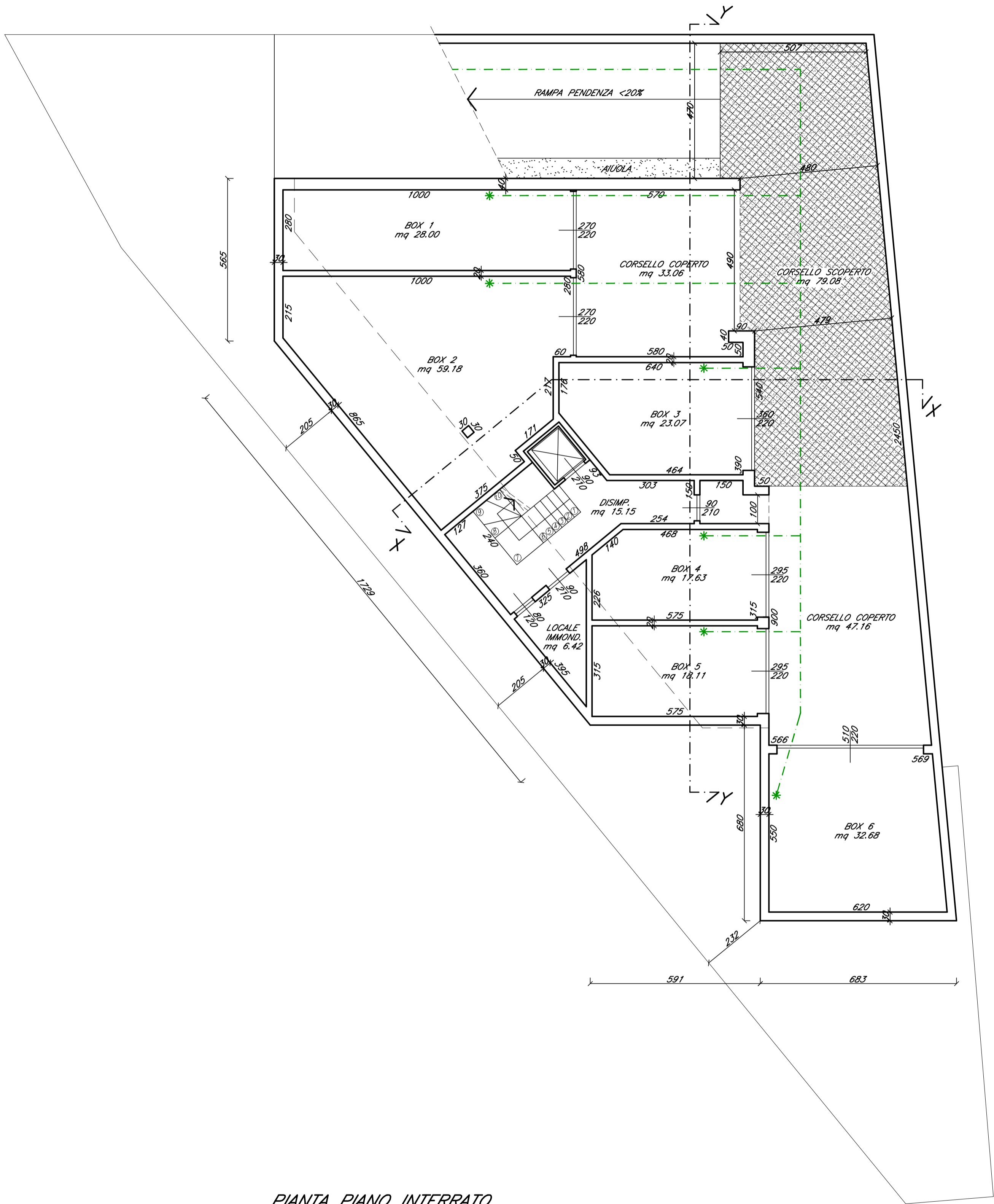
PIANTA PIANO INTERRATO SCALA 1:100
